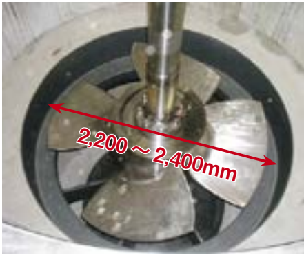
ポンプの羽根車
