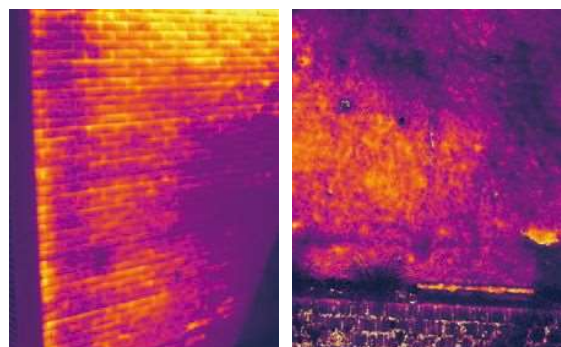
赤外線カメラによる 建物の外壁点検
